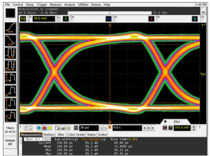
Рисунок 2. Сигнал проходит через активный согласующий адаптер N7010A. Отметим, что какой-либо дополнительный шум отсутствует
