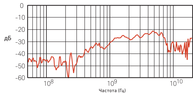
Зависимость коэффициента подавления в синфазном режиме от частоты
