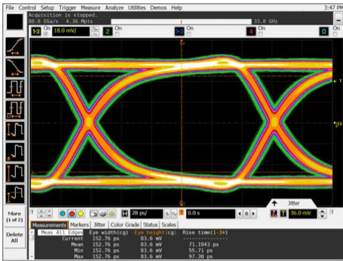
Рисунок 1. Непосредственное подключение сигнала к осциллографу Infiniium
