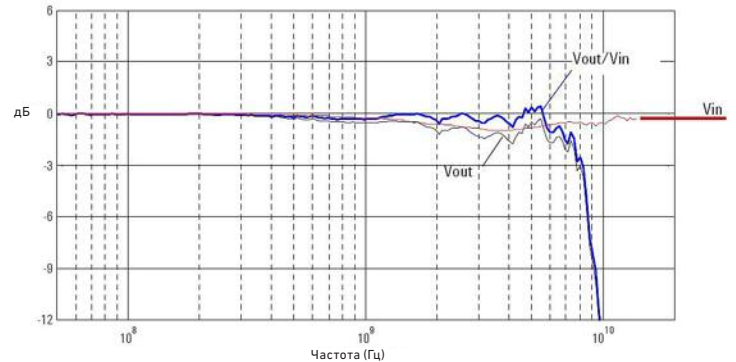
Характеристика качающейся частоты при сопротивлении источника 25 Ом
