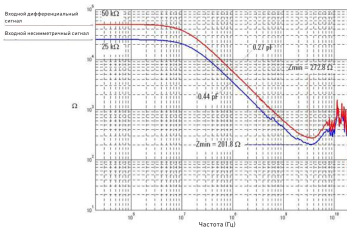
Зависимость входного импеданса от частоты
