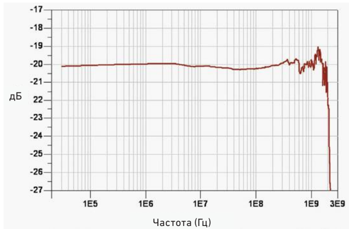
Частотная характеристика пробника N2796A ( V_{out}/V_{in} )
